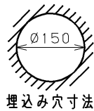
埋込み寸法
