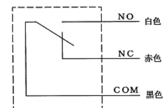
結 線 図
