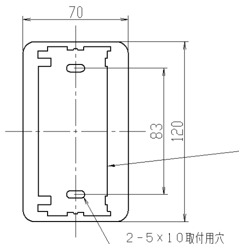
取付寸法（矢視 ①）
