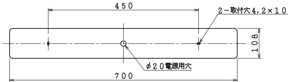
取付寸法(矢視 ①)
