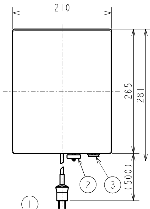
矢視 ㊶ →
