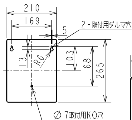
取付寸法(矢視 ①)
