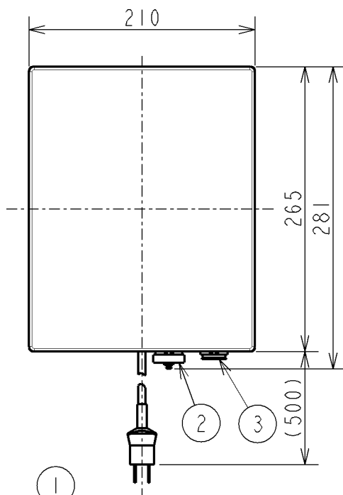
矢視 ② →
