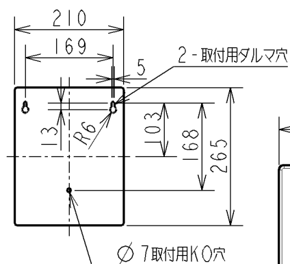
取付寸法 (矢視 ㊦)
