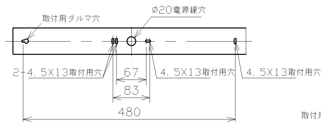
取付寸法
