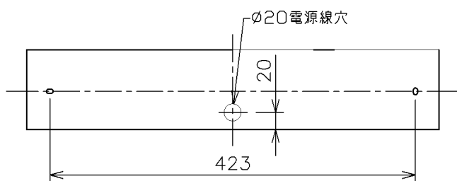
天井取付寸法 (矢視 ⑥)
