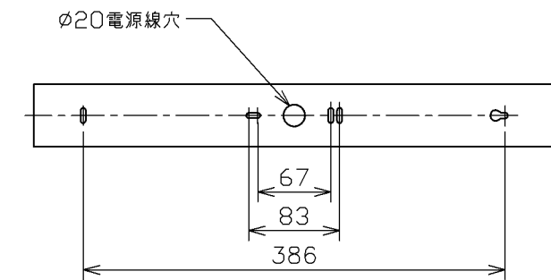
壁取付寸法 (矢視 ④)
