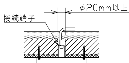
取付寸法 (矢視①)
