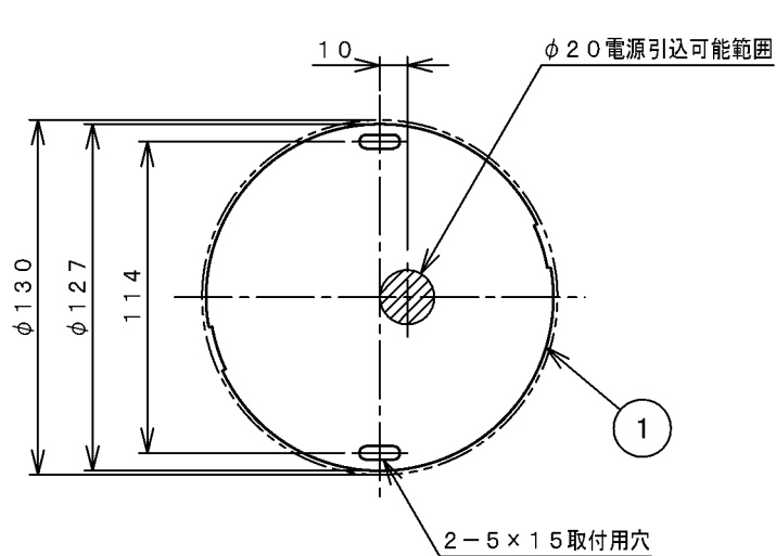
取付寸法（矢視 a）
