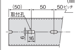
取付孔(底面)寸法図 (mm)
