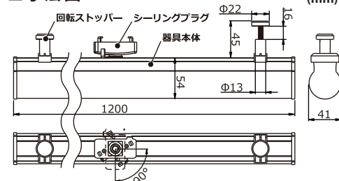
■寸法図
