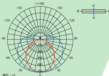
■配光図
